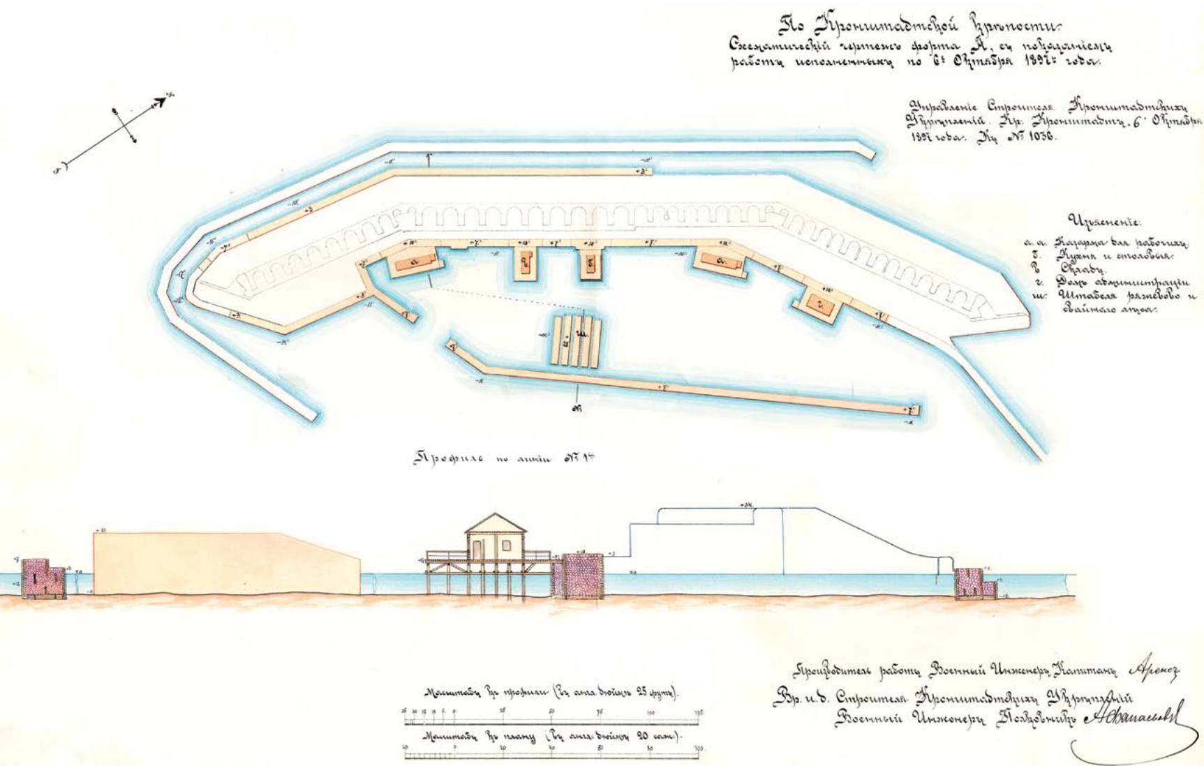
План форта Тотлебен с демонстрацией работ, выполненных к 6 октября 1897 г.
