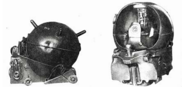
Якорная гальваноударная мина образца 1908 г. Якорная ударно-механическая мина образца 1912 г.
