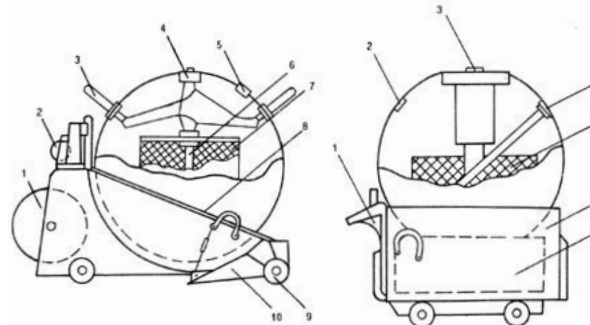
Устройство мины образца 1908 г. 1 - вьюшка с минрепом; 2 - груз шпёрта; 3 - гальваноударный котлаж; 4 - предохранительный прибор; 5 - прибор потопления; 6 - запальное устройство; 7 - зарядная камера; 8 - якорь-тележка; 9 - роульс; 10 - лапа якоря
